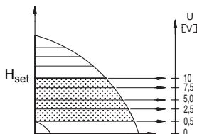
Рис. 3 Пример внешнего регулирования насоса по постоянному давлению с помощью аналогового сигнала 0-10 В
